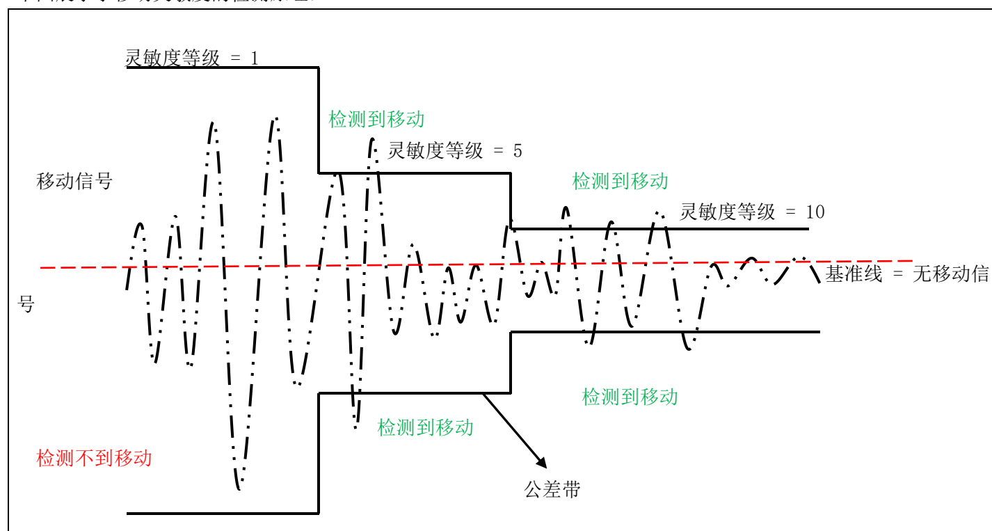
图 4：移动灵敏度
